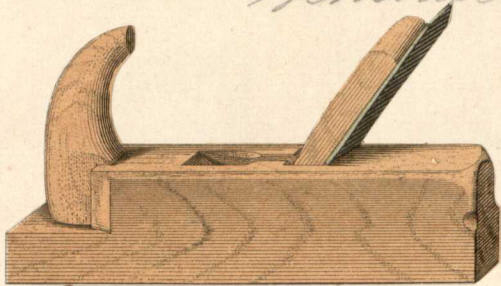
Cepo de plaina e ferros dobrados
